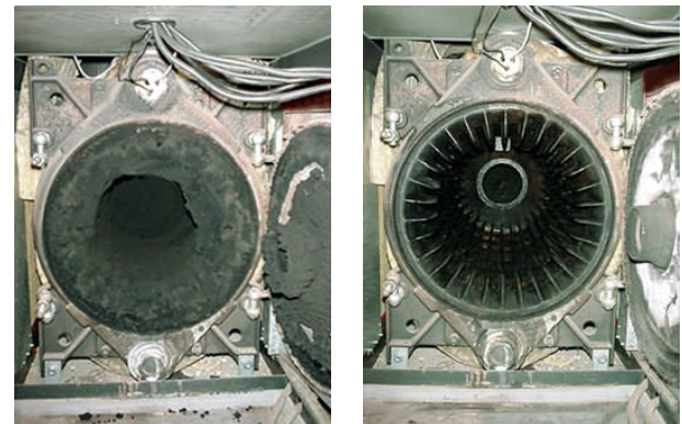
Vergleich: Kessel vor und nach der Reinigung
